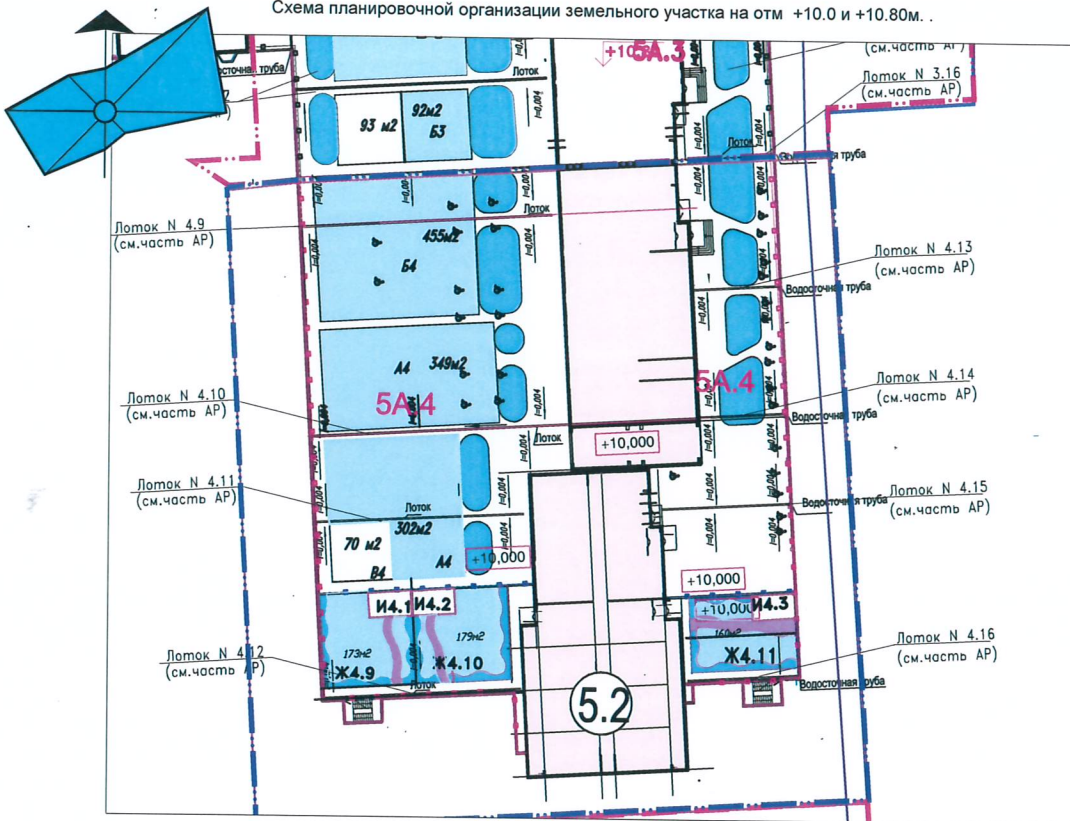
Схема планировочной организации земельного участка на отм +10.0 и +10.80м.
